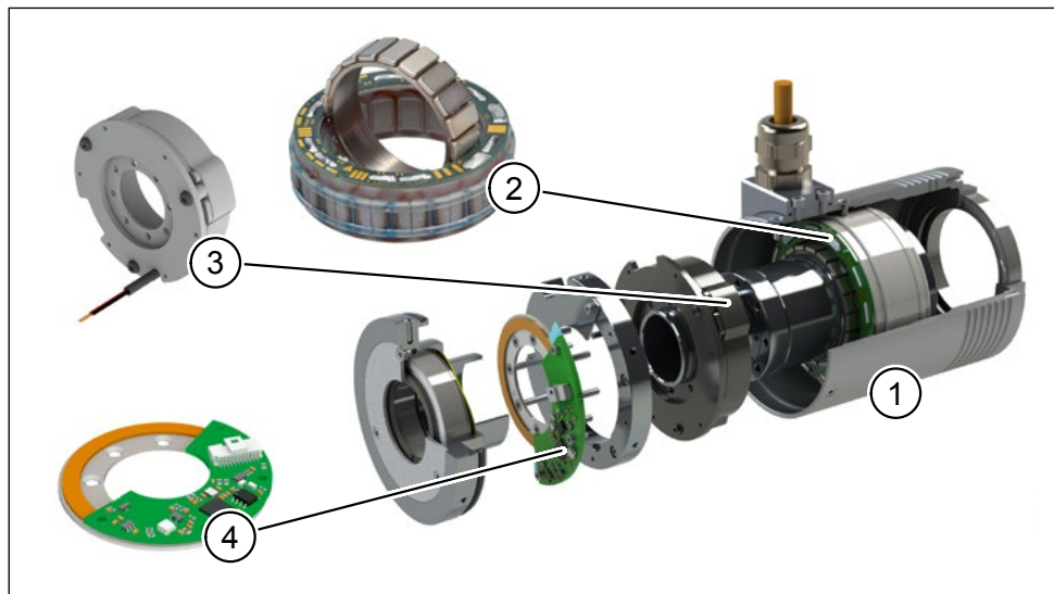
Abb. 2: Beispiel mit Systemkomponenten für Hohlwellenmotor
