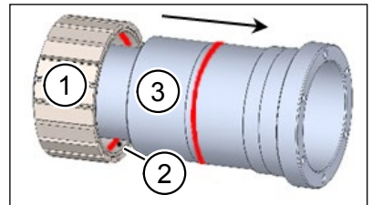
Abb. 15: Rotor auf Welle aufschieben
