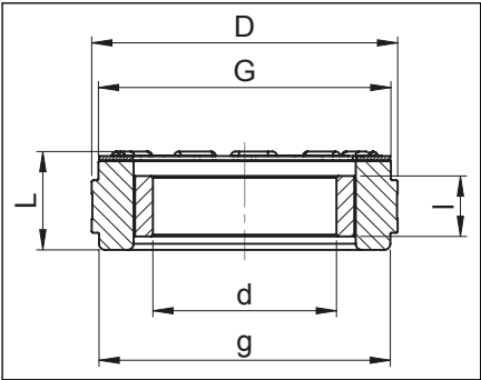
Abb. 5: Maßbezeichnungen
