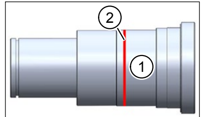
Abb. 13: Klebstoffring auf Welle
