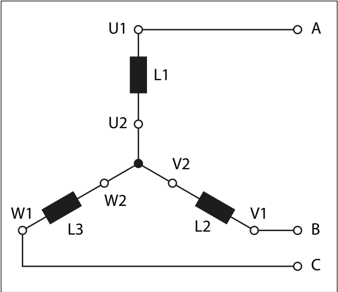
Abb. 4: Messpunkte am ILM Servo-Kit (Verschaltung Stern-seriell)
