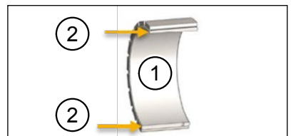
Abb. 16: Druckpunkte am Innenring
