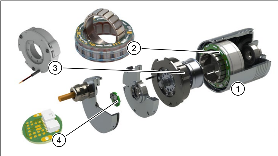
Abb. 3: Beispiel mit Systemkomponenten für Vollwellenmotor
