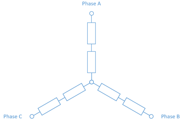
Star-serial
