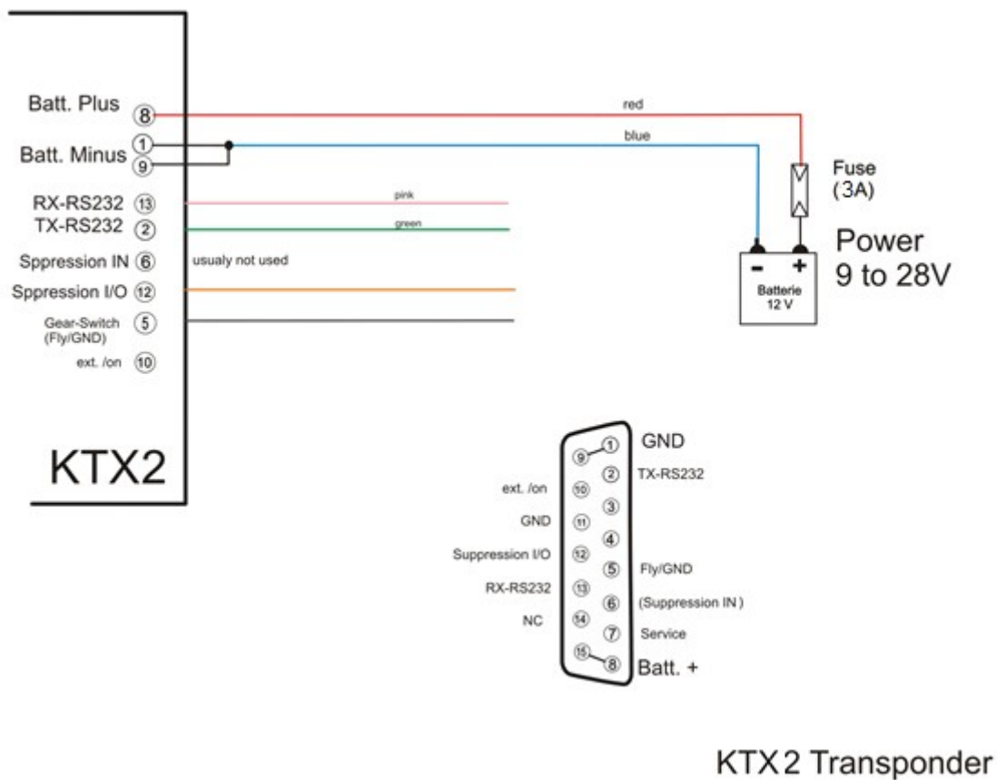
Abbildung 7: Anschlussplan
