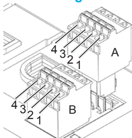
Fig. 4: Schema dei collegamenti per connettore a spina RS485
