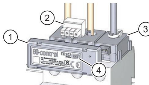
Afb. 5: Sensorbar op stroomsensoren steken
