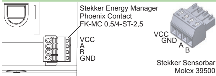
Afb. 4: Bekabeling van de Sensorbar naar de Energy Manager
